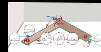
01 Сборка первой «ёлочки»
