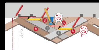
05 Сборка верхнего угла, укладка
