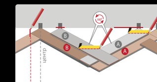
04 Сборка верхнего угла
