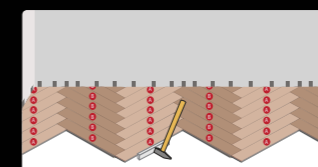
06 Монтаж последующих рядов
